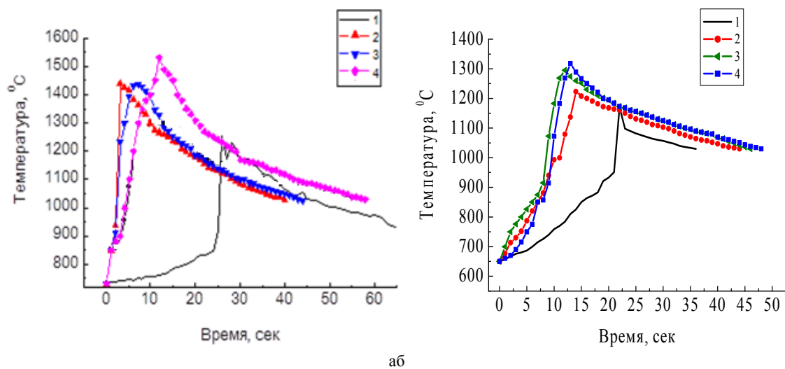
Рисунок 6 - Термограммы горения систем (\text{SiO}_2 + \text{Me}) с алюминием и магнием в исходном состоянии и после 20 минут МХО с разным количеством графита: а - \text{SiO}_2 + (\text{Al}/\text{C}) , б - \text{SiO}_2 + (\text{Mg}/\text{C}) ; 1 - Меисх; 2 - 5 %; 3 - 10 %; 4 - 20 % C
