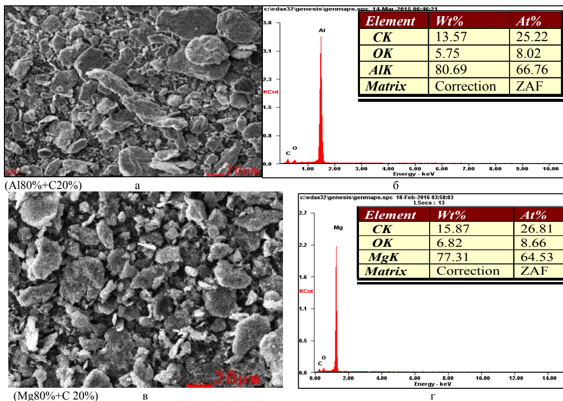
Рисунок 2 - Электронно-микроскопические снимки (а, в), энергодисперсионный спектр и массовая доля элементов (б, г) в композите (Al80%+C 20%) и (Mg 80%+C20%) после 20 минут МХО
